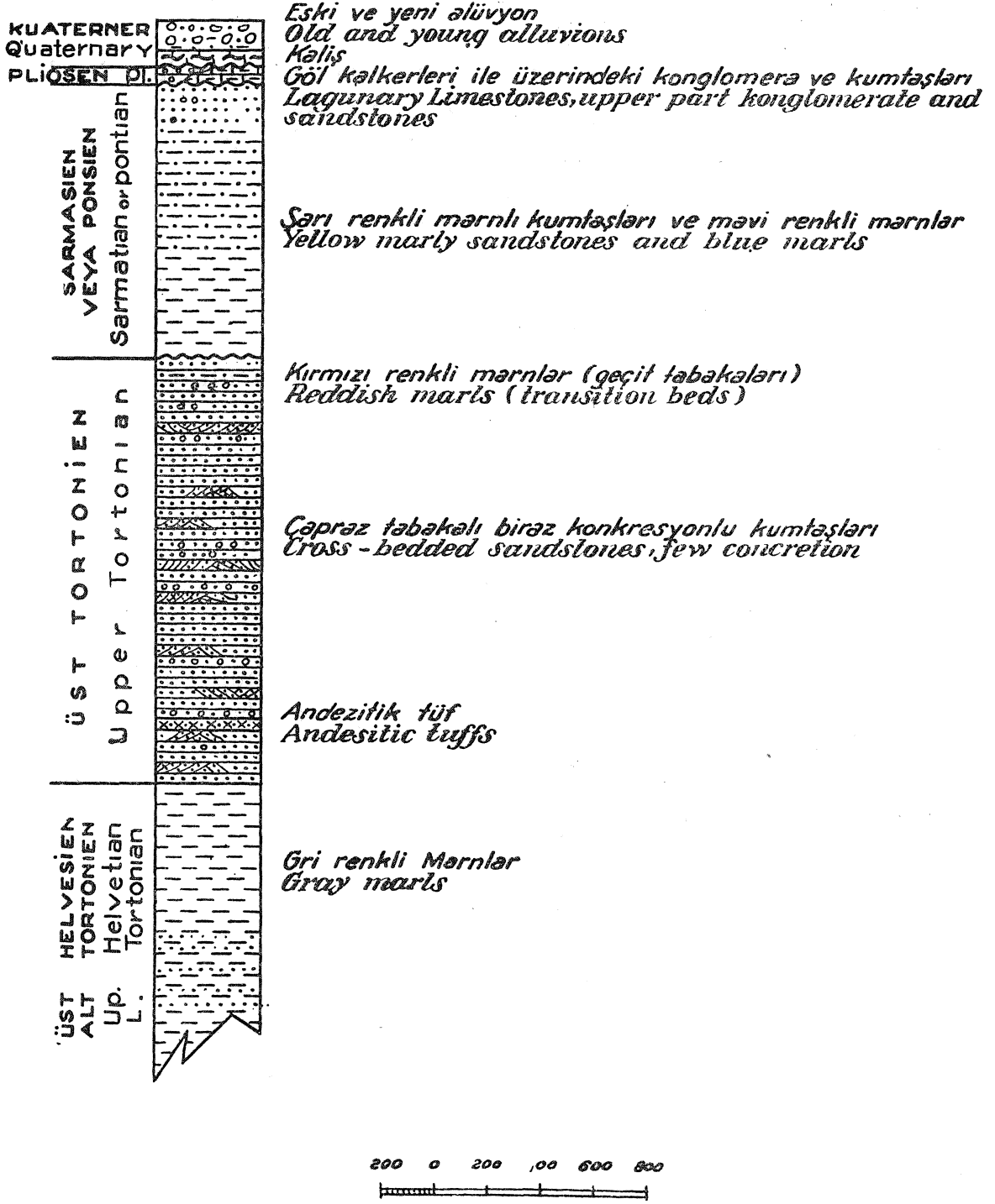
Levha III — BUĞU - KILBAŞ (ADANA) BÖLGESİNİN STRATİGRAFİK DİKİNE KESİŐİ
